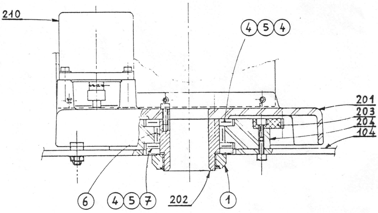
Figure 5: AXE 1 : Base du robot "YOUPI"
